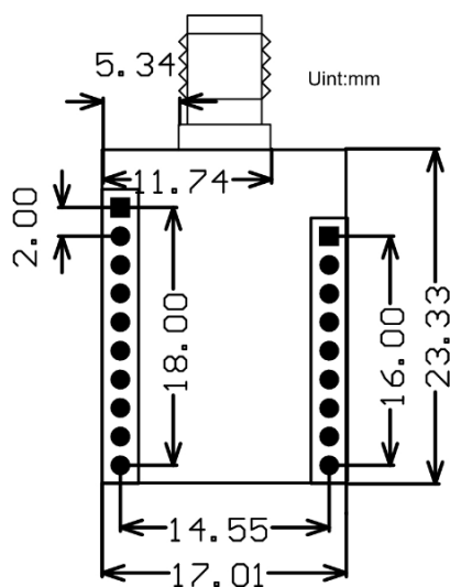
图 1-2 WLT2408NZ 结构尺寸
