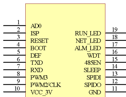
图 1-4 模块引脚排列图
